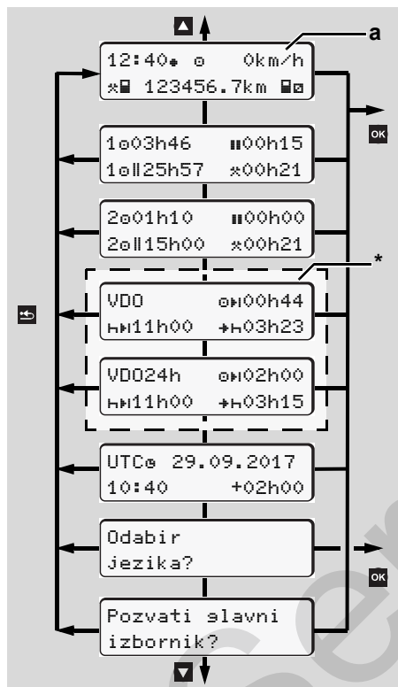
Upravljanje u prvoj ravni menija
